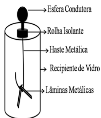
Fig- 11. Electrôscópio de folha
