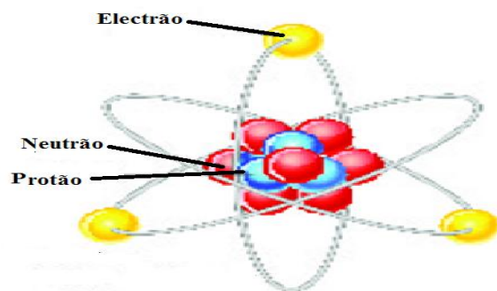
Fig. 1- Os protões e neutrões estão ligados dentro do núcleo por forças nucleares fortes.
