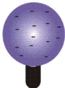
Fig.8 – Corpo induzido já carregado negativamente
