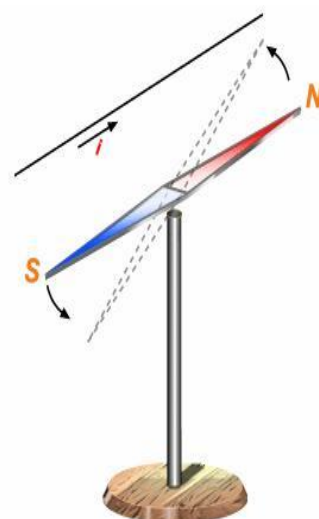
Fig.1 – Uma agulha magnética girando e indicando os pólos magnéticos do íman.
