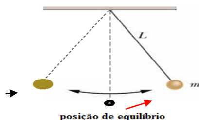
Fig. 1B - Pêndulo Simples.
