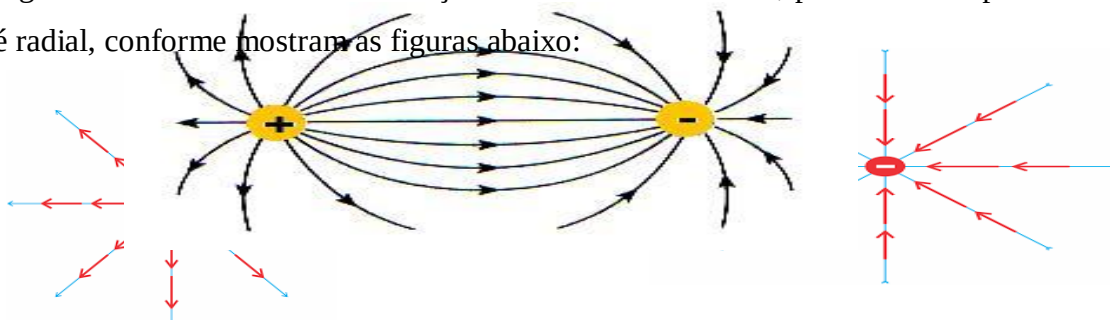
Fig. 11B- linhas de forças são convergentes
