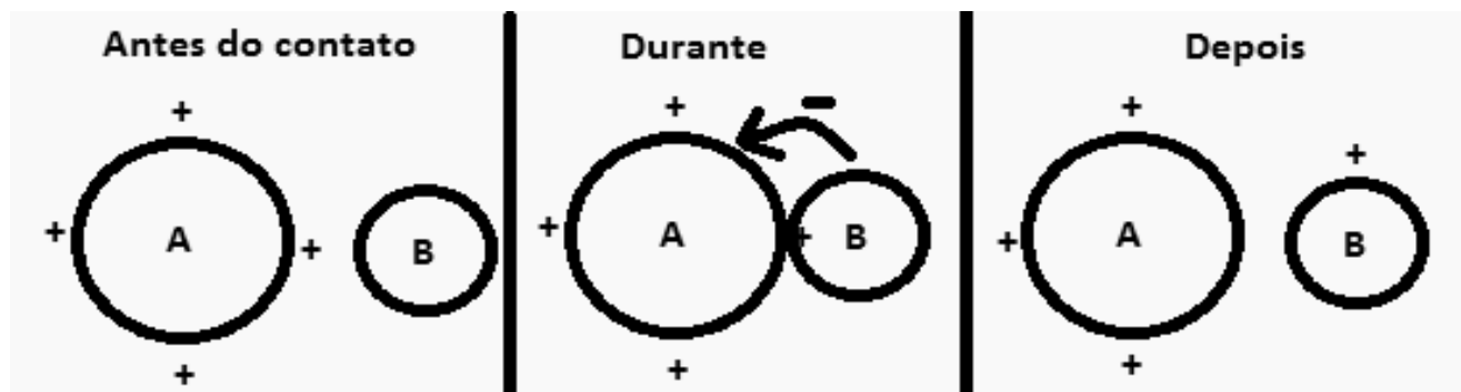
Fig.5 - Electrização por contacto
