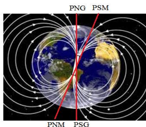
Fig. 7 Linhas do campo magnético da terra, em que PNM é o pólo norte magnético, PSM, pólo sul magnético, PPSG, pólo norte geográfico e PSG, pólo sul geográfico.
