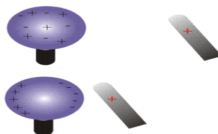
Fig.6 – Bastão electrizado aproximado ao induzido
