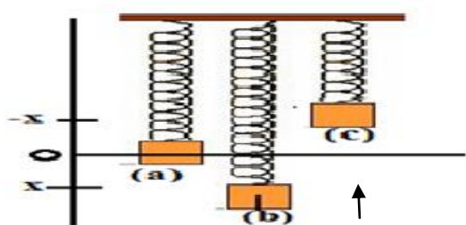
Fig. 1A- Mola em vibração (Pêndulo elástico).
