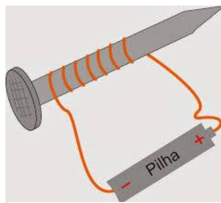
Fig. 10 Exemplo de electroíman
