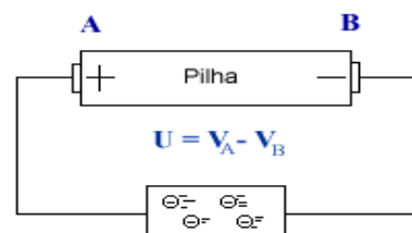
Fig.14 – Uma pilha conectado em paralelo e ele serve como fonte da tensão.
