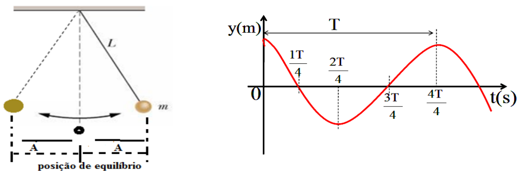
Fig. 3 - Pêndulo Simples e o gráfico que descreve o movimento oscilatório do pêndulo ao lado.
