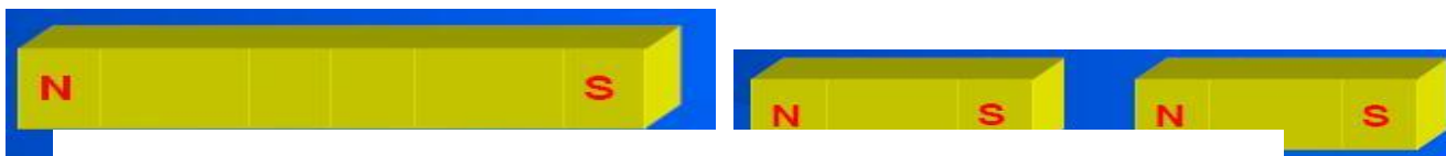
Fig. 2- íman dividida em duas partes iguais e gera imanes com dois pólos de dois nomes diferentes.
