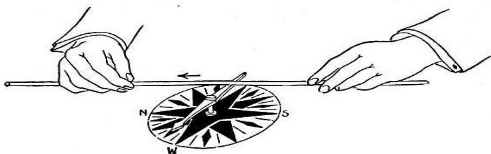
Fig. 7 A agulha metálica da bússola sai da posição paralela ao fio para uma posição perpendicular, quando há corrente atravessando o fio.
