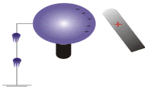
Fig.7 – Corpo induzido ligado à Terra.
