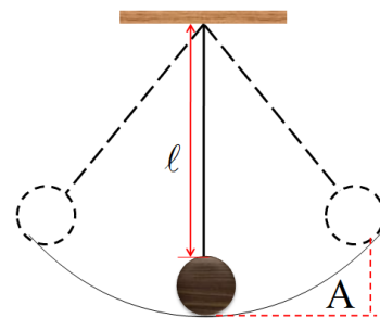
Fig. 4 – Pêndulo simples ou gravítico
