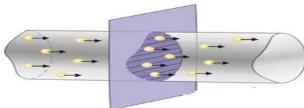
Fig. 12: Electrões atravessando a secção recta de um fio condutor
